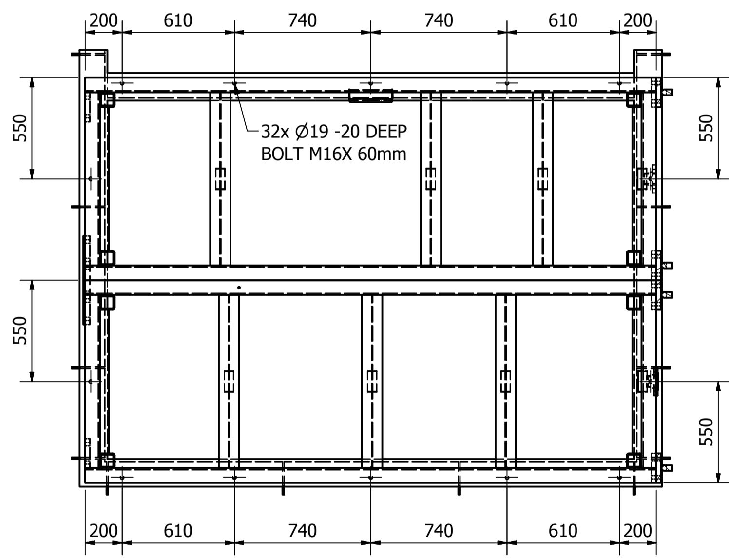
SECTION C-C ( 1 : 20 )
